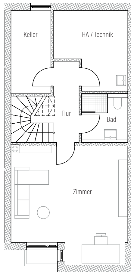
Basisgeschoss
